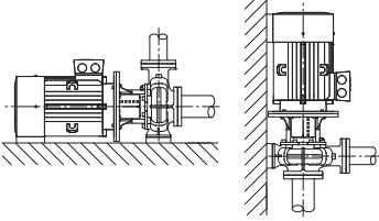
Fig. 5: Atmos GIGA-B görünümü
