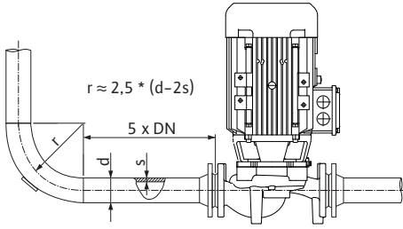
Fig. 13: Pompadan önce ve pompadan sonra sönümlenme hattı
