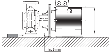
Pompa gövdesi destekli, motor temel üzerine sabitlenmiş
