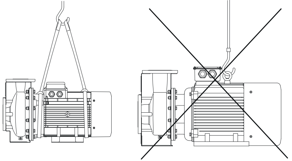
Fig. 1: Pompanın nakliyesi
