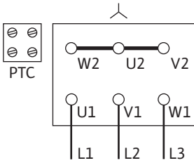
Fig. 7: Y devresi
