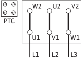
Fig. 6: Δ devresi
