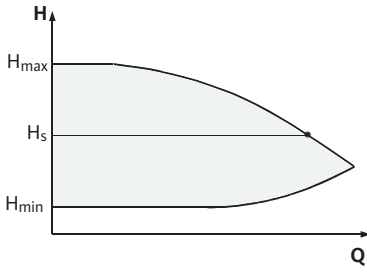
Fig. 6: Kontrol modu \Delta p-c
