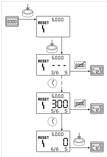
Fig. 58: Hata tipi C'nin onaylanması
