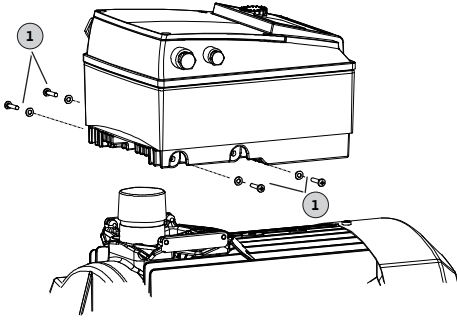
Fig. 48: Elektronik modülün değiştirilmesi
