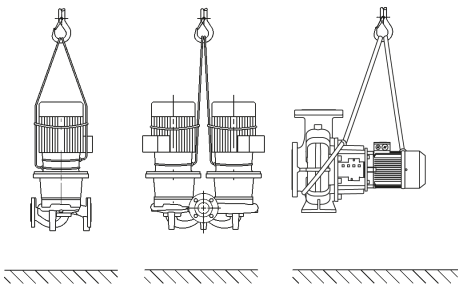
Fig. 1: Pompanın nakliyesi
