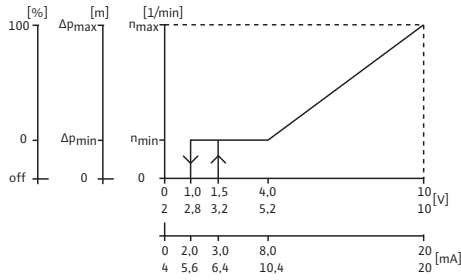
Fig. 12: Giriş ve çıkışların davranış şekli
