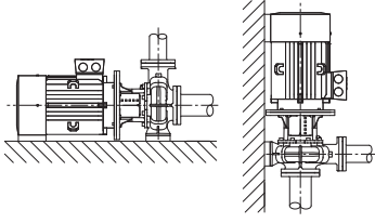
Fig. 4: Atmos GIGA-B görünümü
