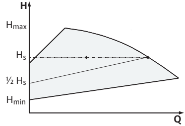
Fig. 7: Kontrol modu \Delta p-v
