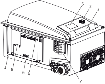
Fig. 5: Elektronik modül, genel bakış
