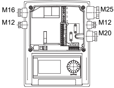
Fig. 29: Kablo bağlantıları
