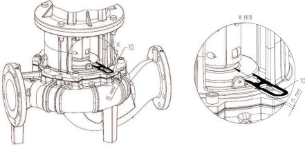
Fig. 47: Montaj çatalının yerleştirilmesi
