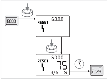
Fig. 55: Hata tipi B'nin onaylanması ( X < Y )
