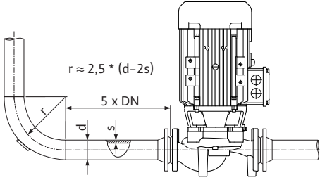
Fig. 18: Pompadan önce ve pompadan sonra sönümleme hattı
