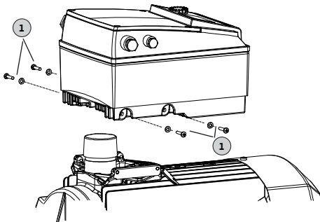
Fig. 49: Elektronik modül – motor bağlantısı
