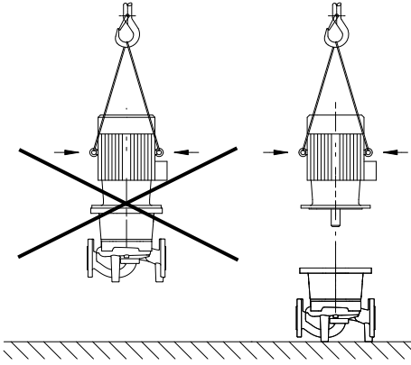
Fig. 2: Motorun nakliyesi
