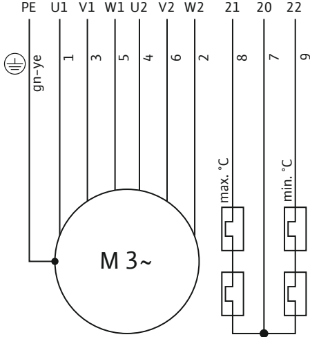
Fig. 6: 3~ motor bağlantı şeması: Yıldız üçgen açma devresi, bimetal sensör
