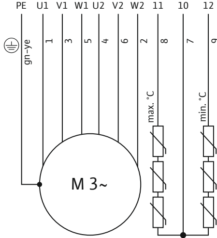
Fig. 7: 3~ motor bağlantı şeması: Yıldız üçgen açma devresi, PTC sensör
