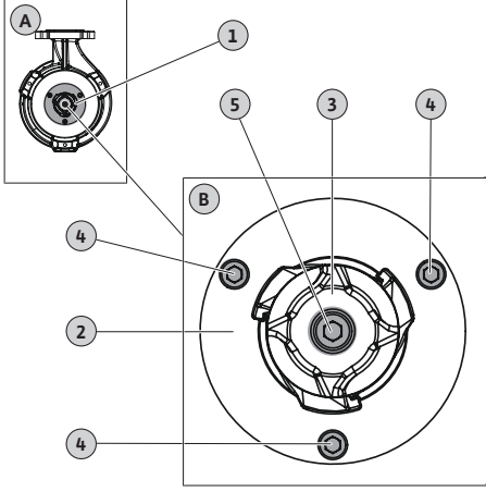
Fig. 9: Parçalayıcı bıçak değişimi
