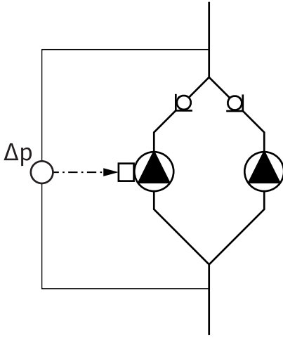
Fig. 9: Örnek - Birleştirme parçası kurulumunda fark basıncı sensörünün bağlantısı
